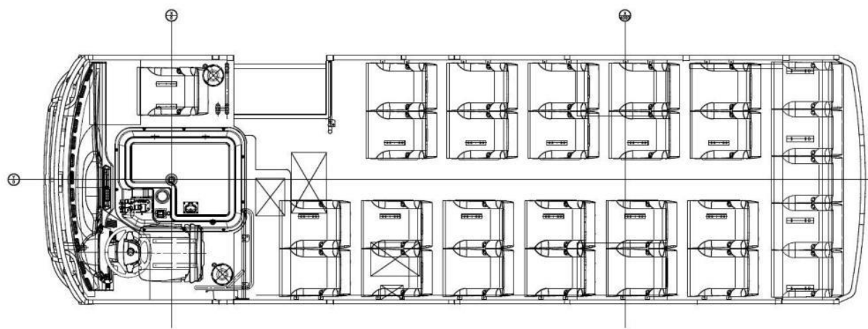
نمودار چیدمان صندلی برای مدل فرمان چپ BJ ۶۷۳۰ (تعداد صندلی: ۲۹)
