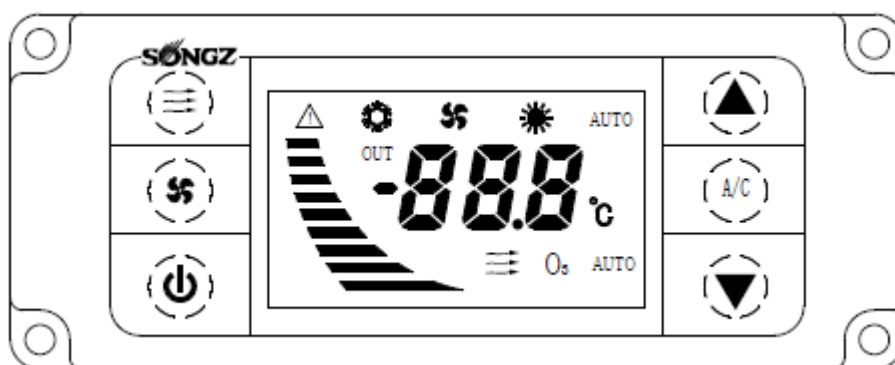
شکل ۴-۱: پنل کنترل A/C (صفحه نمایش LED)
