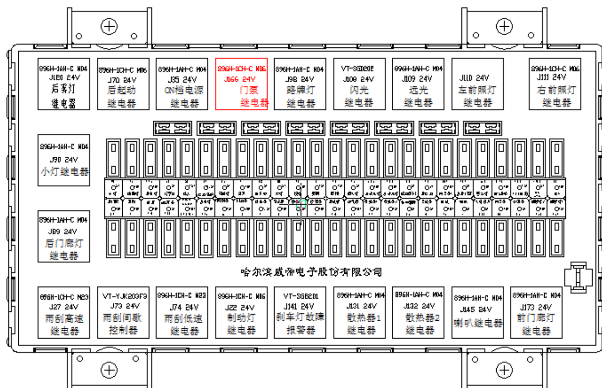
شكل ۳-۳۳: جعبه فیوز
